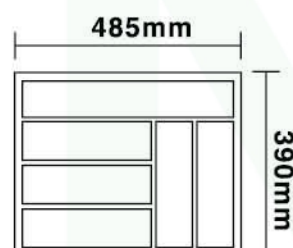
刀叉盘 Knife and fork holder 型号 Item: K-804S (白色 / 灰色)
