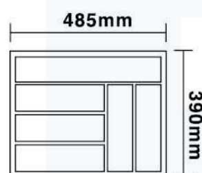
刀叉盘 Knife and fork holder 型号 Item: K-804H (白色 / 灰色)
