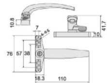
CA811 七字执手
