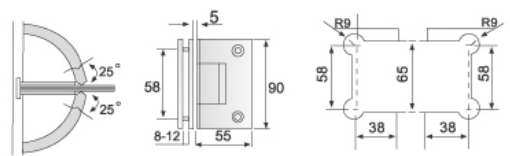
V-90D 90° 双面直边
