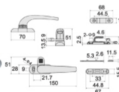
CA866 七字执手
