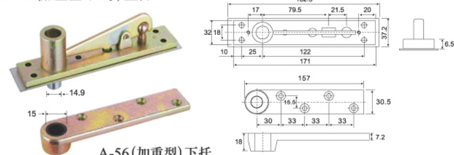
A-56(加重型6厘厚) 上托
