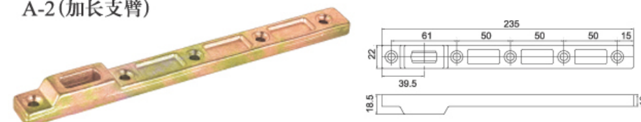
A-2(加长支臂)
