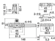
CA844 七字执手
