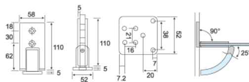
SD-032 90° 单边长夹
