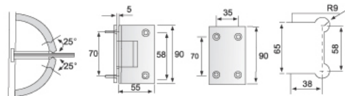
S-90A 90° 双边直边
