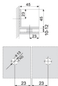
SD-04 90° 斜边
