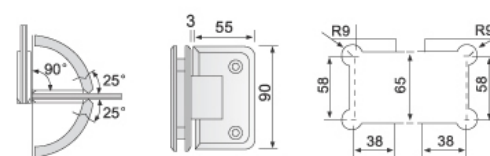
SD-90D 90° 双面斜边
