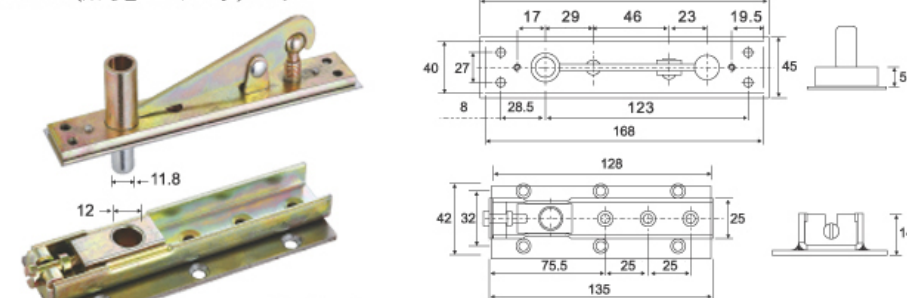
A-56(加宽型) 下托
