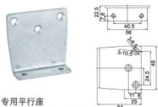
专用平行座 Special parallel block
