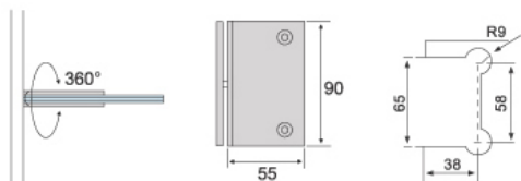
S-9002 360° 直边
