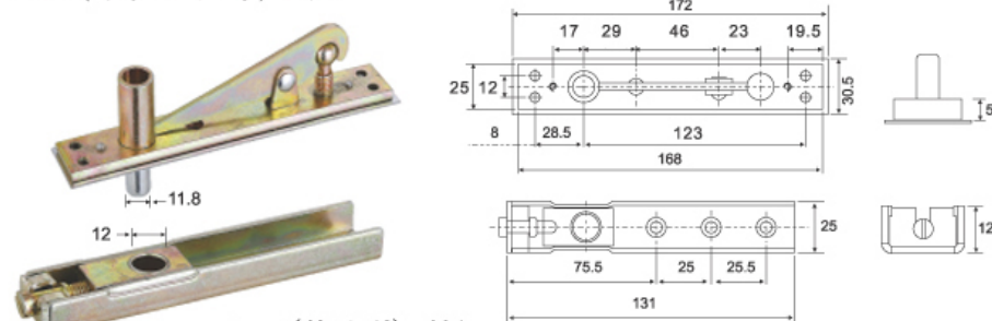
A-56(普及型) 下托
