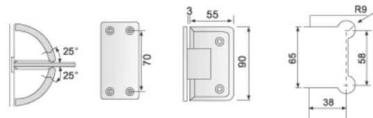
SD-90A 90° 双边斜边
