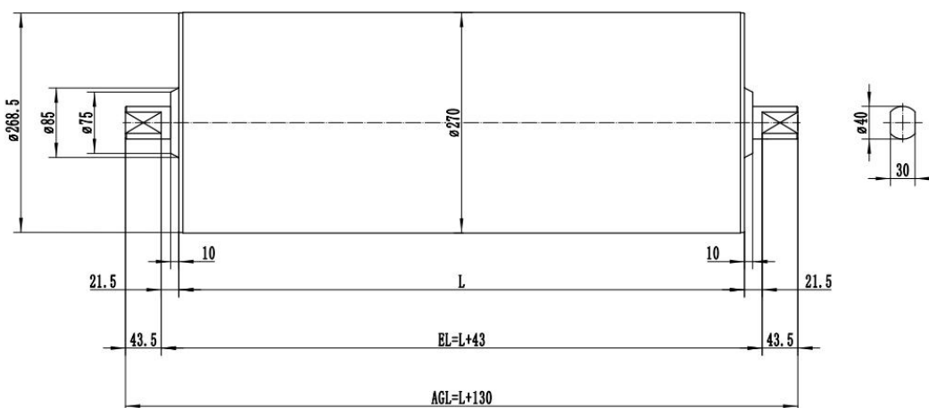
UT270H Idler roller
