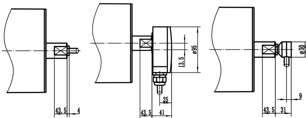
UT270H Idler roller
