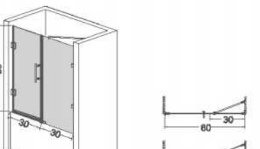
TUB DOOR K-R12T
