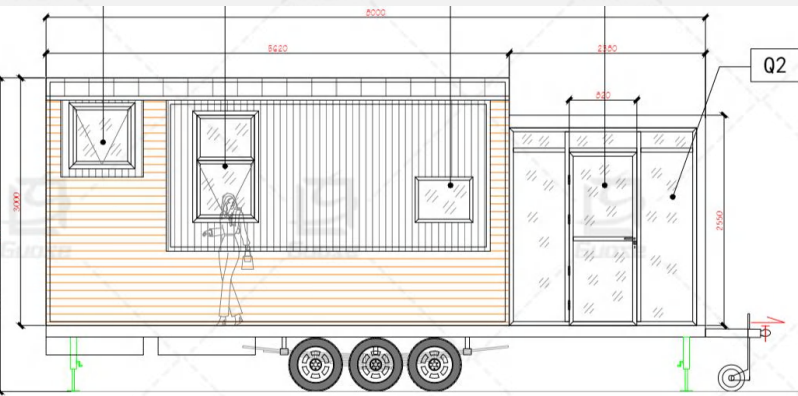
正视图
