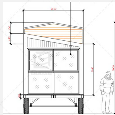
右视图
